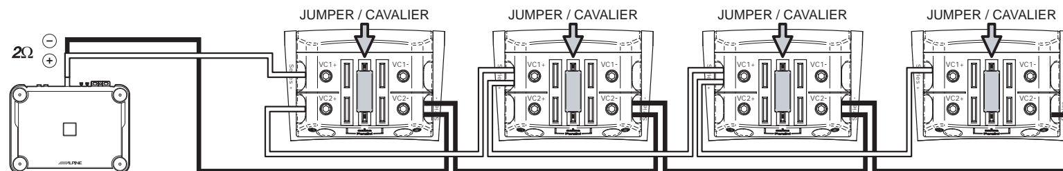
Exemple 6 amplificateur et 4 h.-p. d'extrêmes graves
