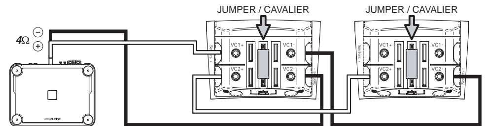
Exemple 4 1 amplificateur et 2 h.-p. d'extrêmes graves
