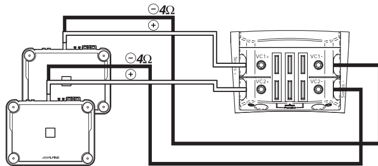
Exemple 3 2 amplificateurs et 1 h.-p. d'extrêmes graves
